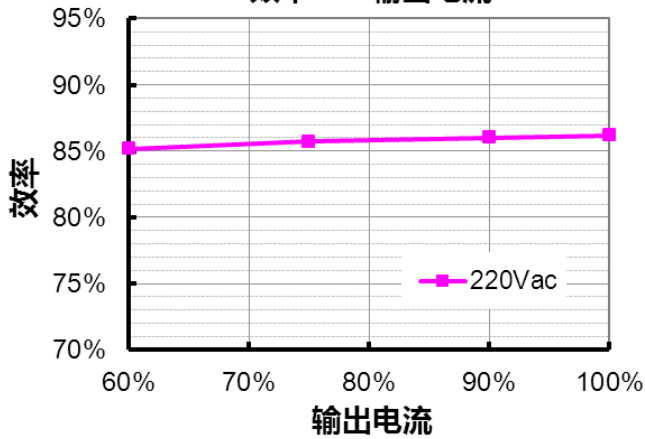
EBV-036S048SVF 效率 vs. 输出电流
