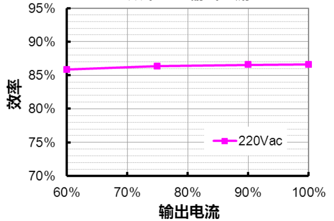
EBV-036S036SVF 效率 vs. 输出电流
