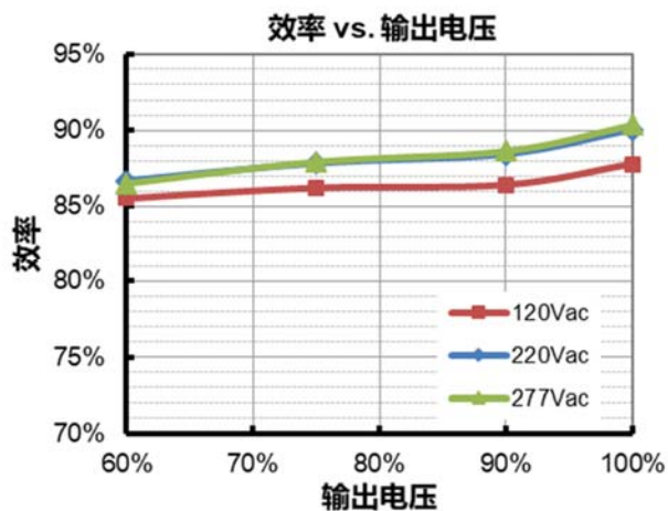
EUM-075S105SV( I_o=1050mA )
