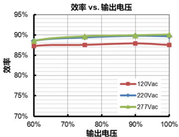
EUM-075S105SV( I_o=700mA )
